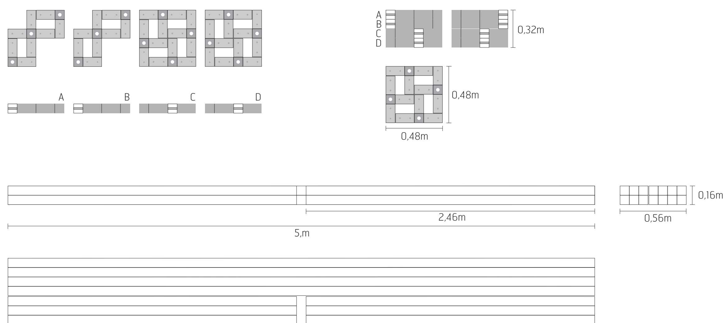
Volumetria para transporte dos componentes Matrix
